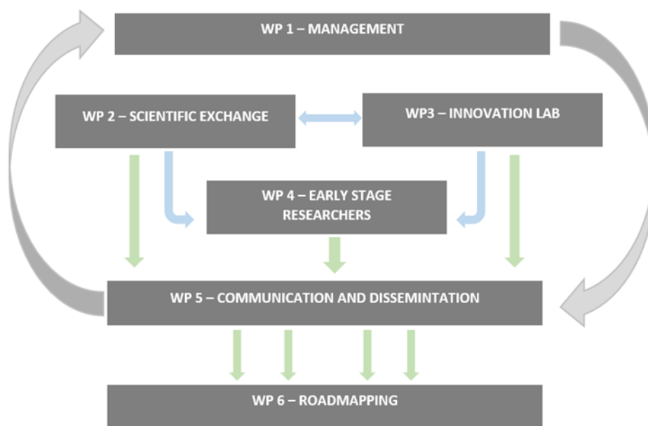
Obrázek 1 Struktura projektu
