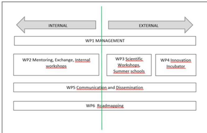
Obrázek 1 Struktura projektu
